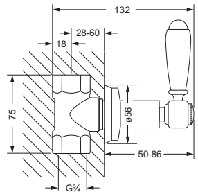
mit Einbaukörper 3/4"
