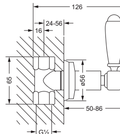
mit Einbaukörper 1/2"
