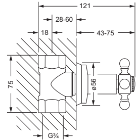
mit Einbaukörper 3/4"
