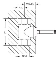
Einbaukörper 3/4"
