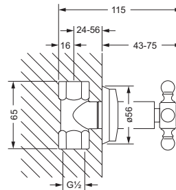
mit Einbaukörper 1/2"
