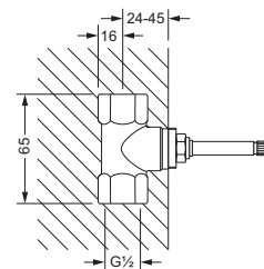
Einbaukörper 1/2"
