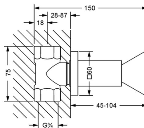
mit Einbaukörper / with concealed body \frac{3}{4} "
