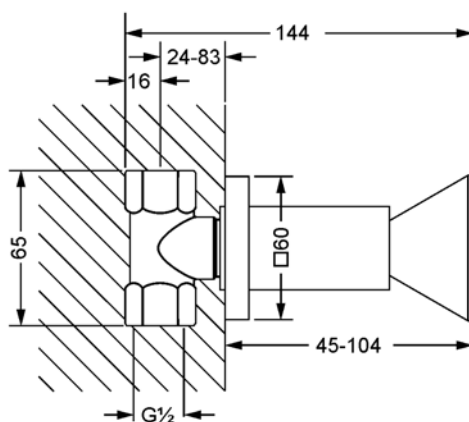
mit Einbaukörper / with concealed body \frac{1}{2} "
