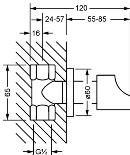
mit Einbaukörper / with concealed body 1/2"
