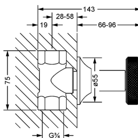
mit Einbaukörper / with concealed body \frac{3}{4} "
