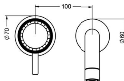
mit Einbaukörper / with concealed body 649.20.364.000
