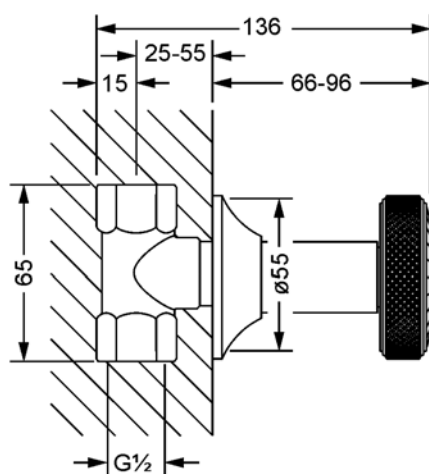
mit Einbaukörper / with concealed body \frac{1}{2} "
