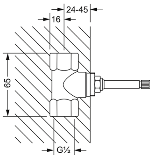
Einbaukörper ½"
