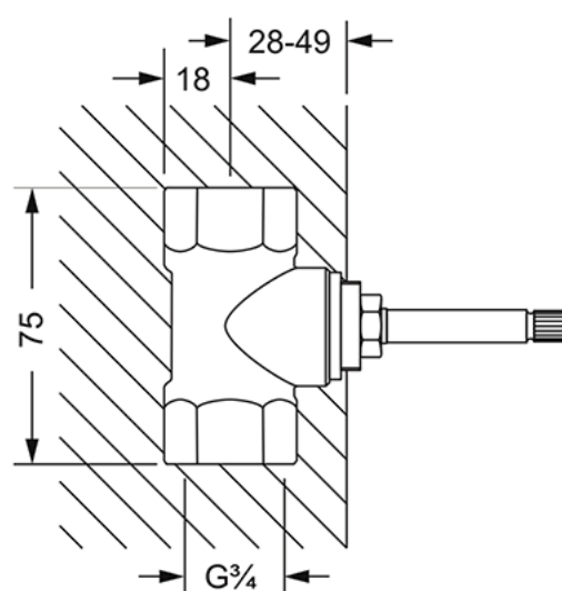
Einbaukörper \frac{3}{4} "
